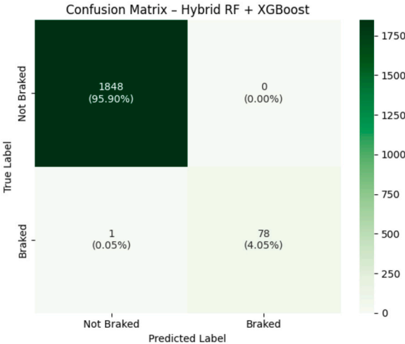
Fig. 17. Confusion Matrix.
