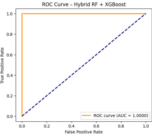
Fig. 15. ROC-AUC Curve.
